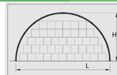
L: 12000 mm Agritunnel H: 6000 mm Arco singolo
